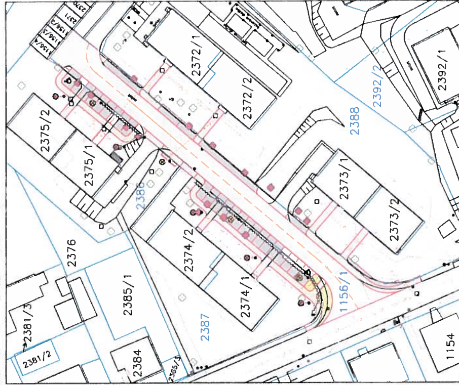
SO 104 CHODNÍKY – NOVÉ ŘEŠENÍ
